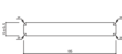
15×105×3,000 (E4E 形状)
