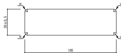
30×105×3,000 (E4E 形状)
