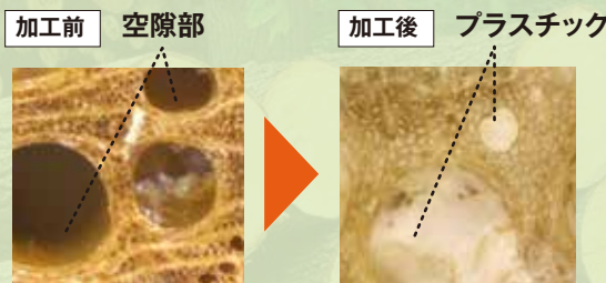
木材のマイクロスコープ断面写真
